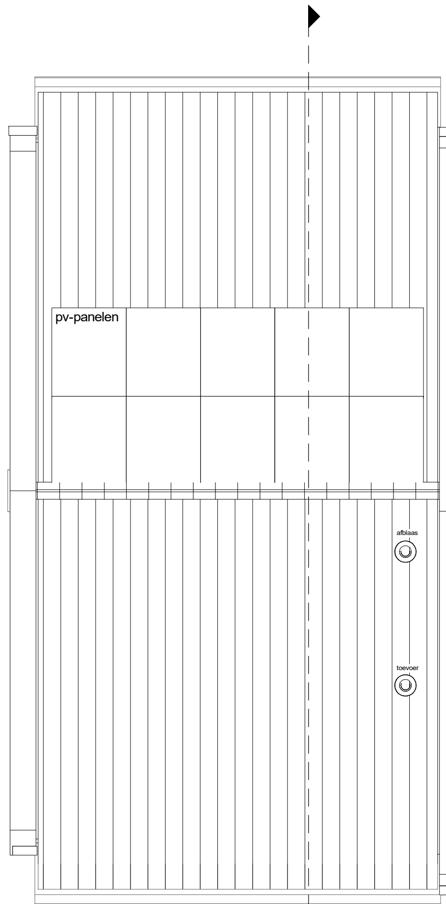
dakaanzicht
