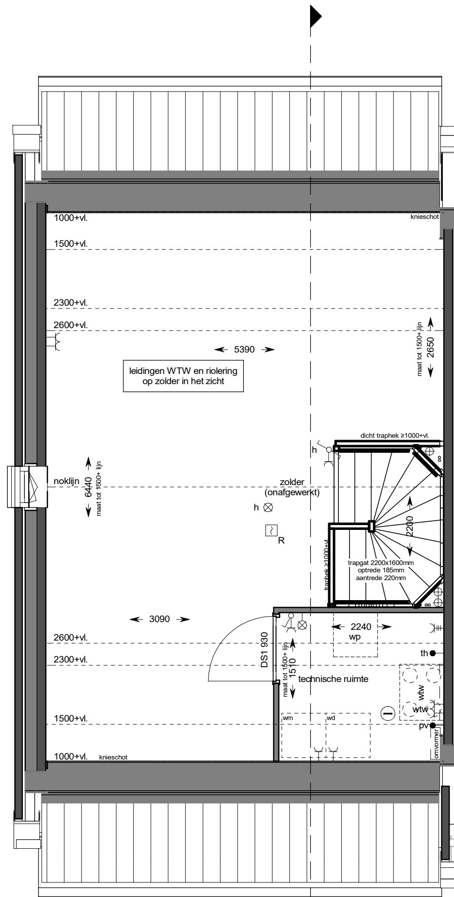
tweede verdieping
