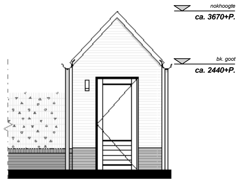
voorgevel
