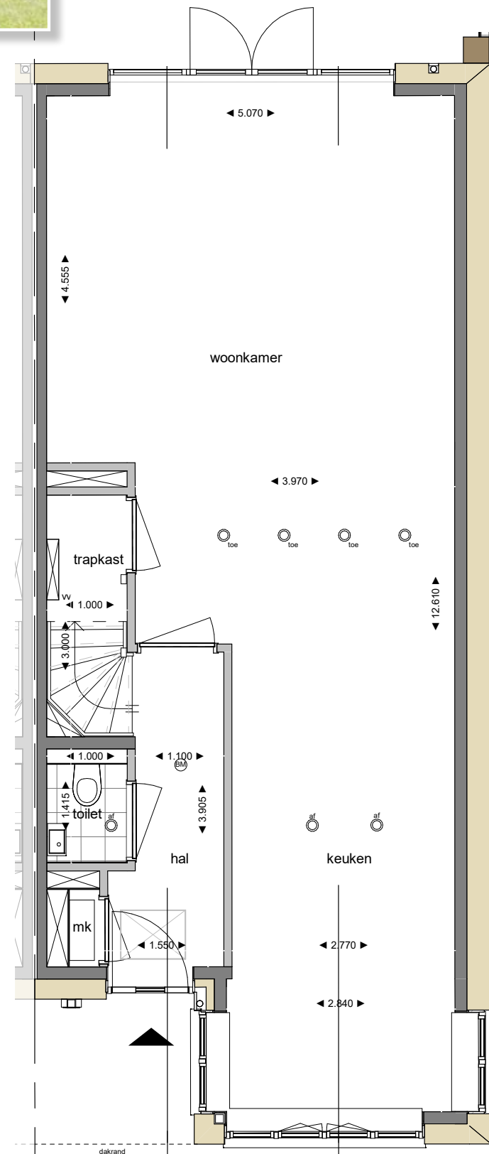
BEGANE GROND
