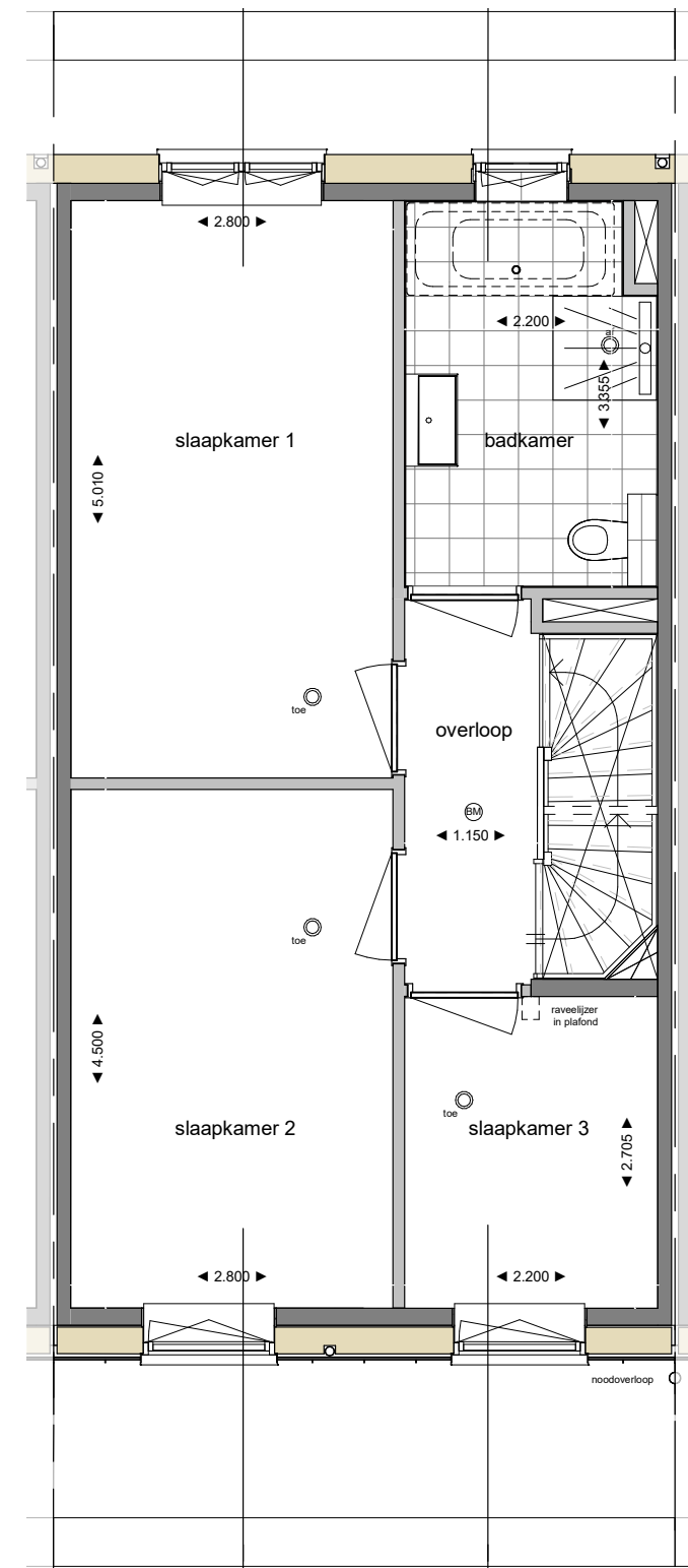
EERSTE VERDIEPING
