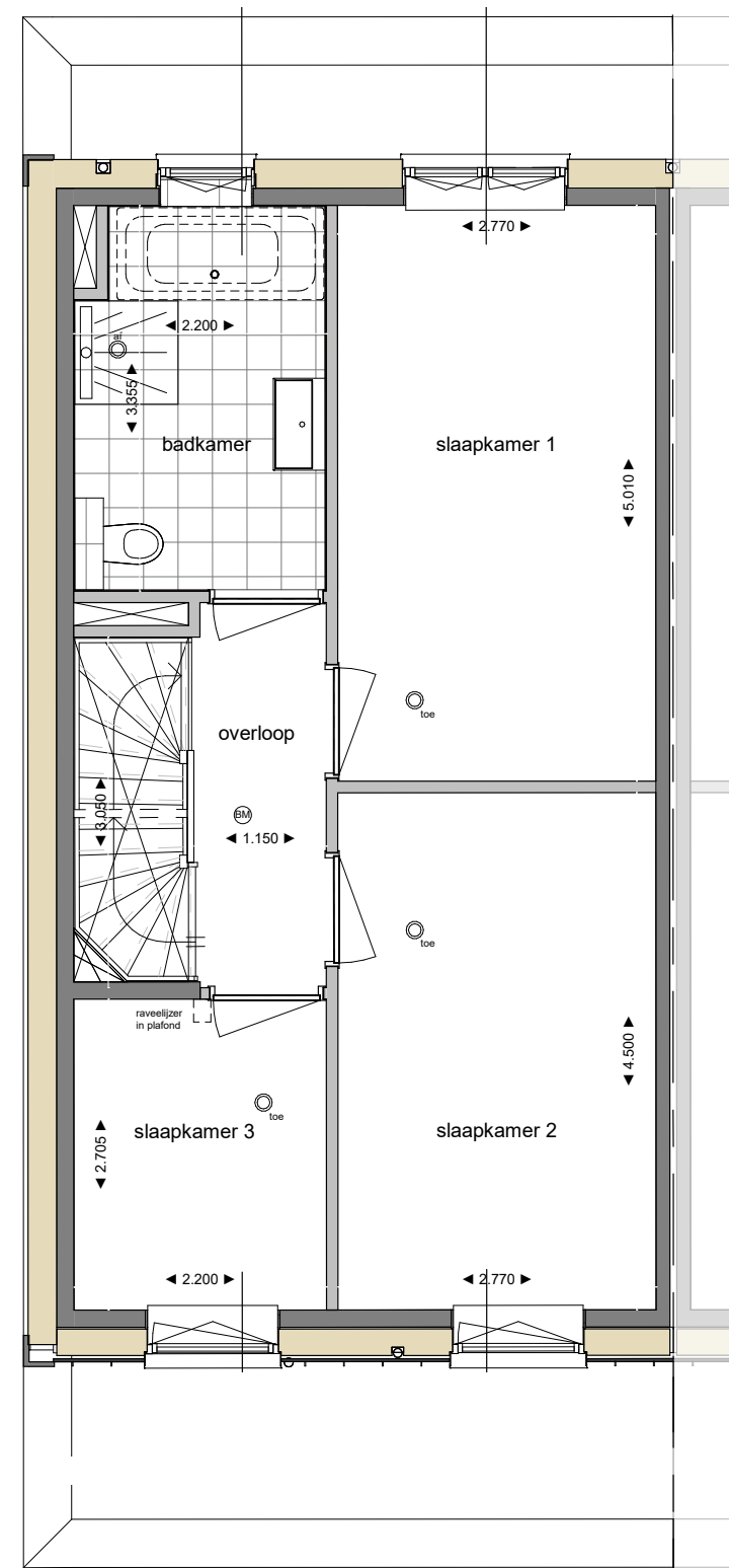
EERSTE VERDIEPING
