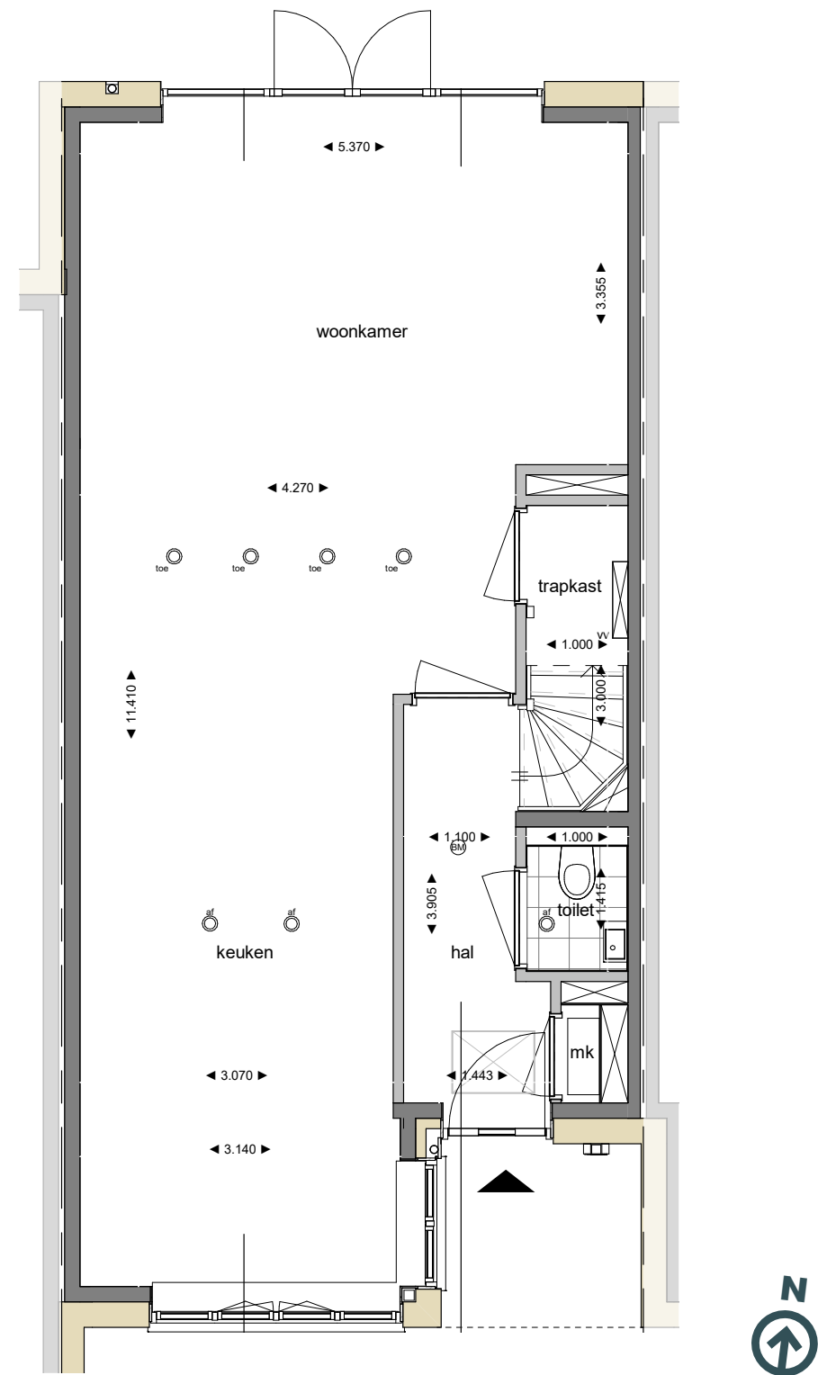
BEGANE GROND
