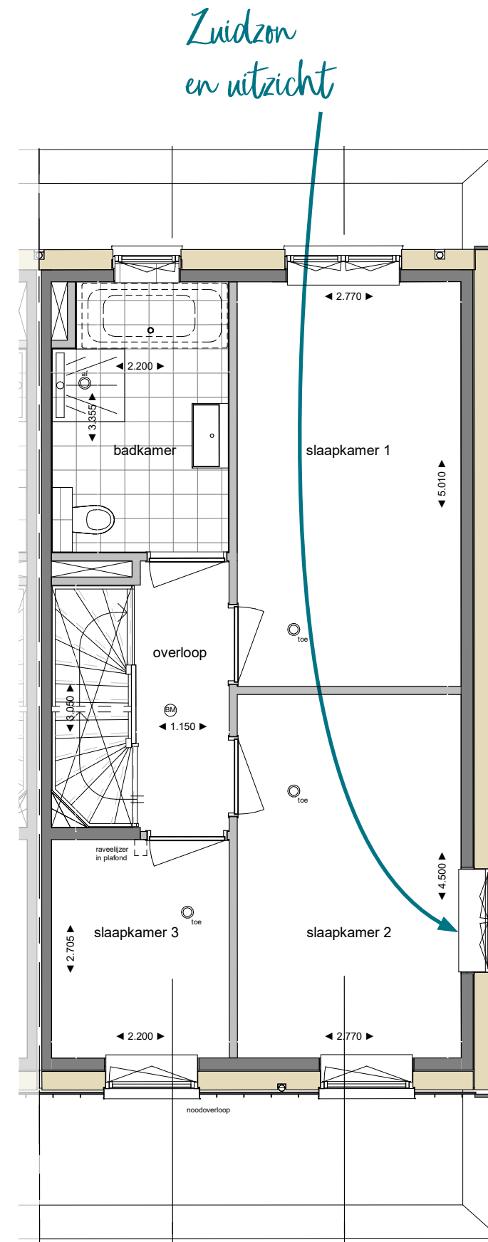
EERSTE VERDIEPING
