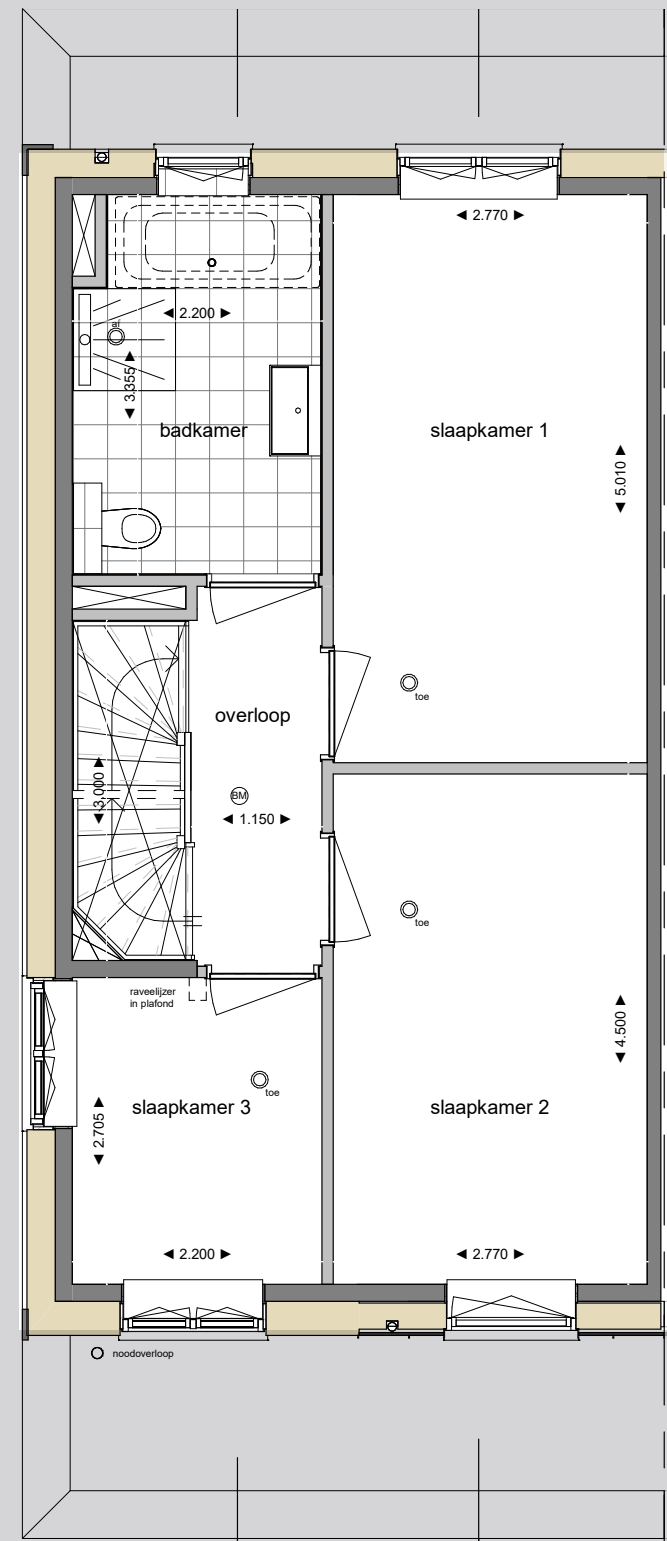
EERSTE VERDIEPING
