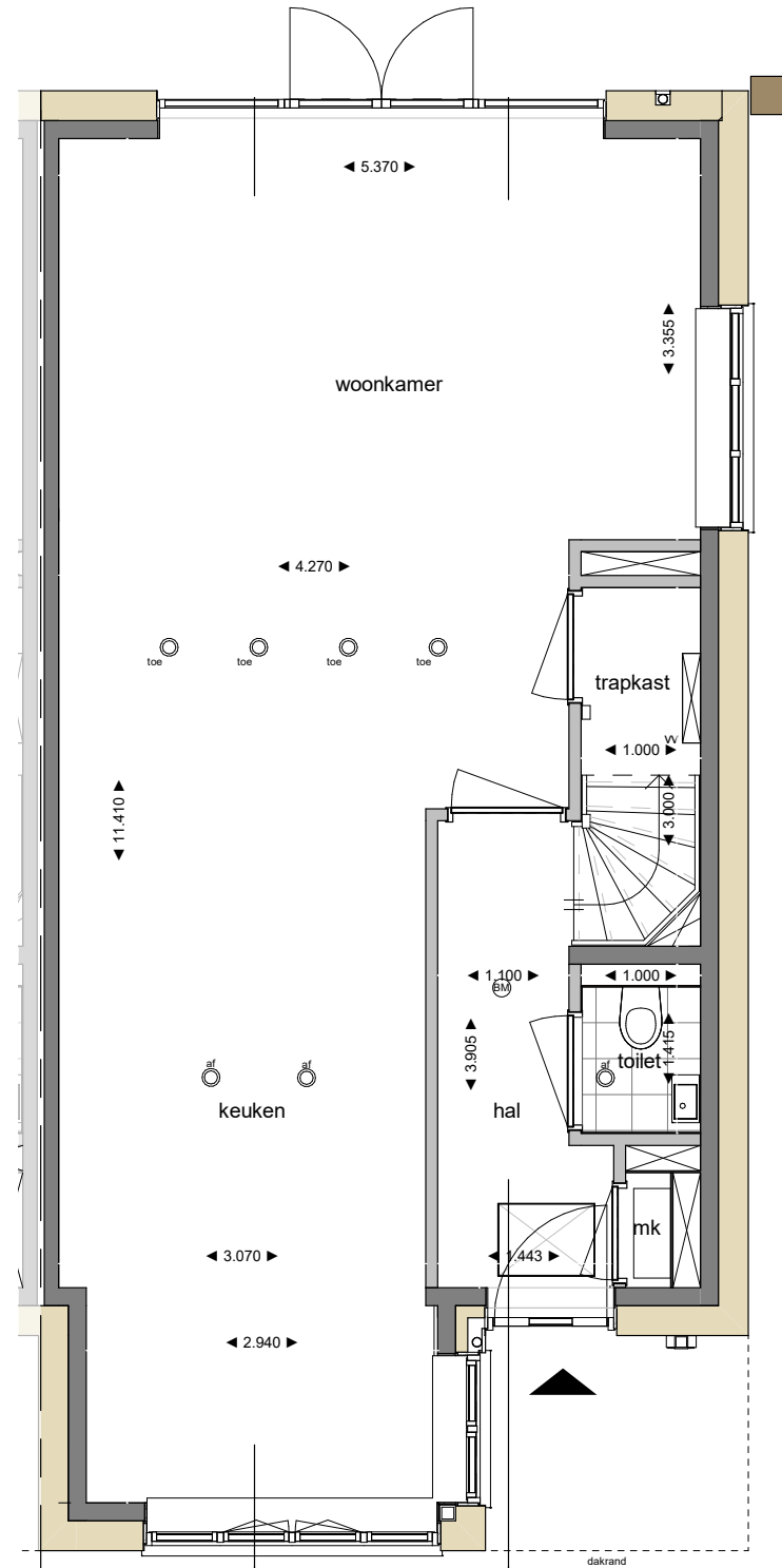
BEGANE GROND
