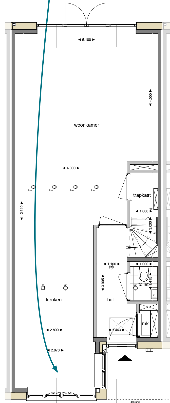
BEGANE GROND
